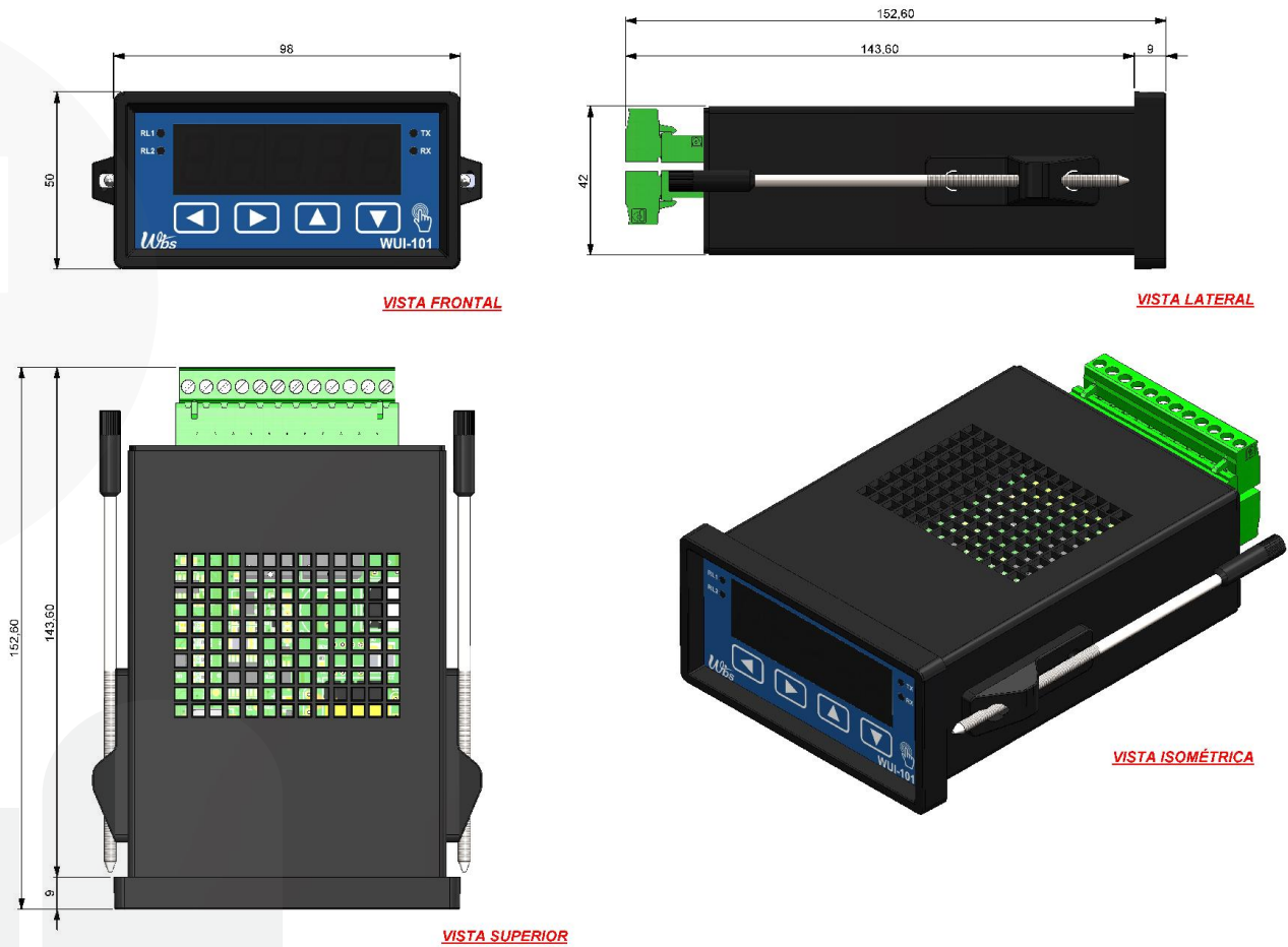
Figura 1 – Dimensionamento para montagem (cotas em milímetro)
