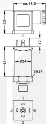
ISO 4400 (IP 65)
